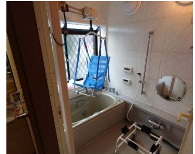
キャリーチェア部吊上げ
