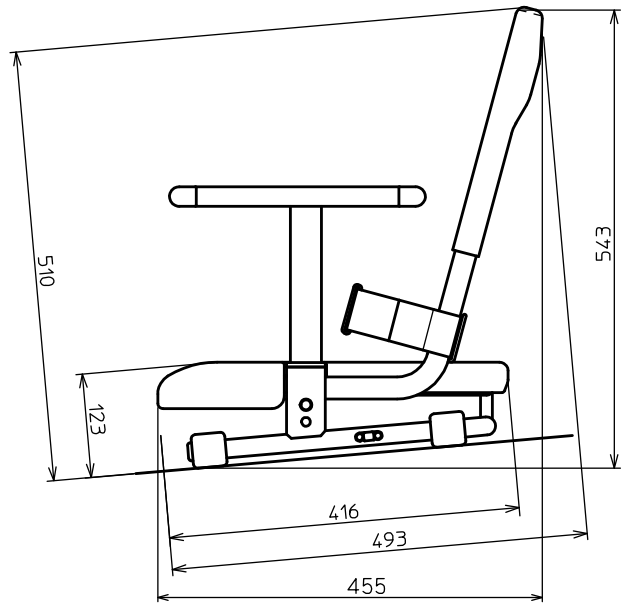
チェア外観寸法
