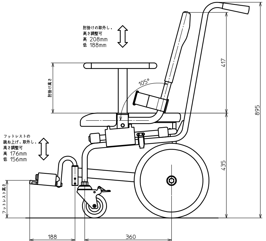
全体外観寸法
